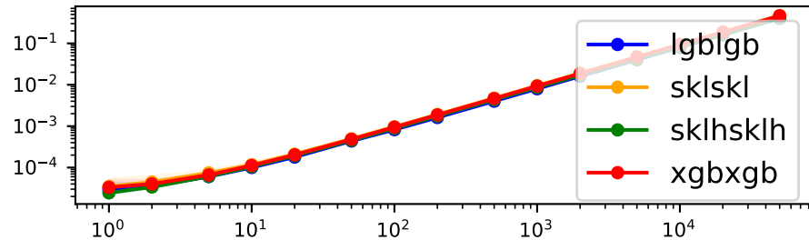
dataset=digits
